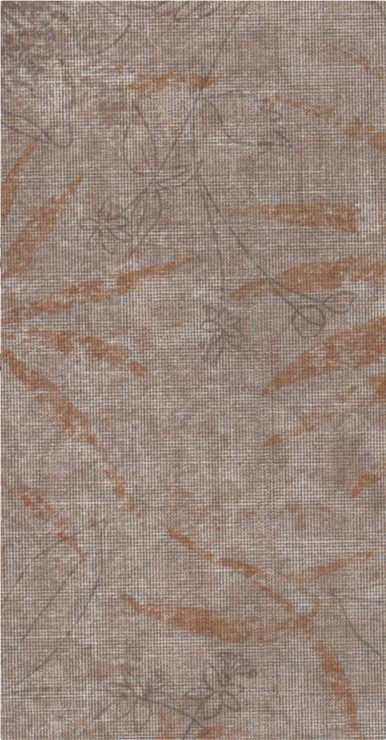
FV | 327
